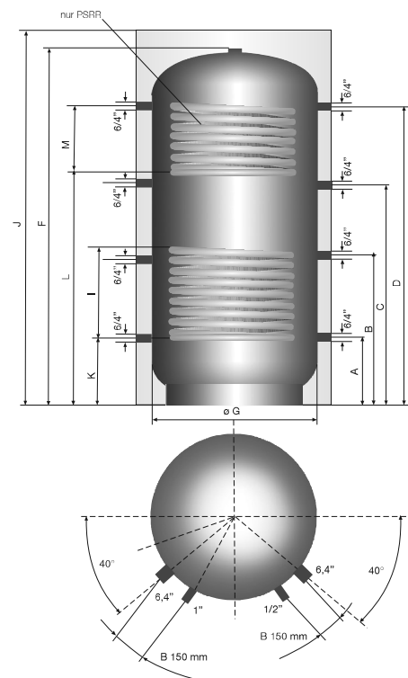
PSR/PSRR PUFFERSPEICHER MIT ROHRREGISTER
